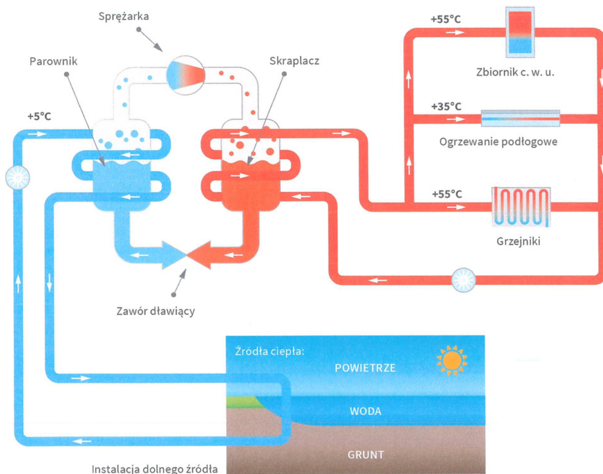
Rys. Ogólny schemat działania pompy ciepła
