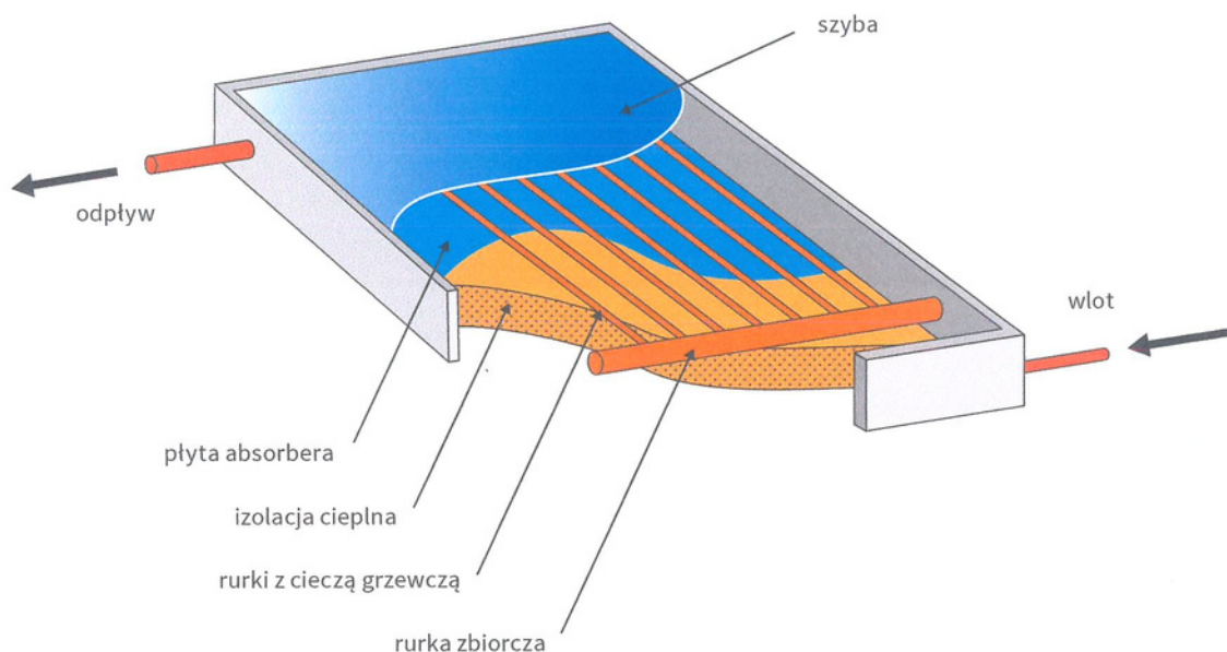
Rys. Budowa kolektora płaskiego
