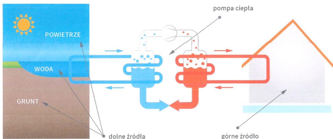
Rys. Dolne i górne źródła ciepła
